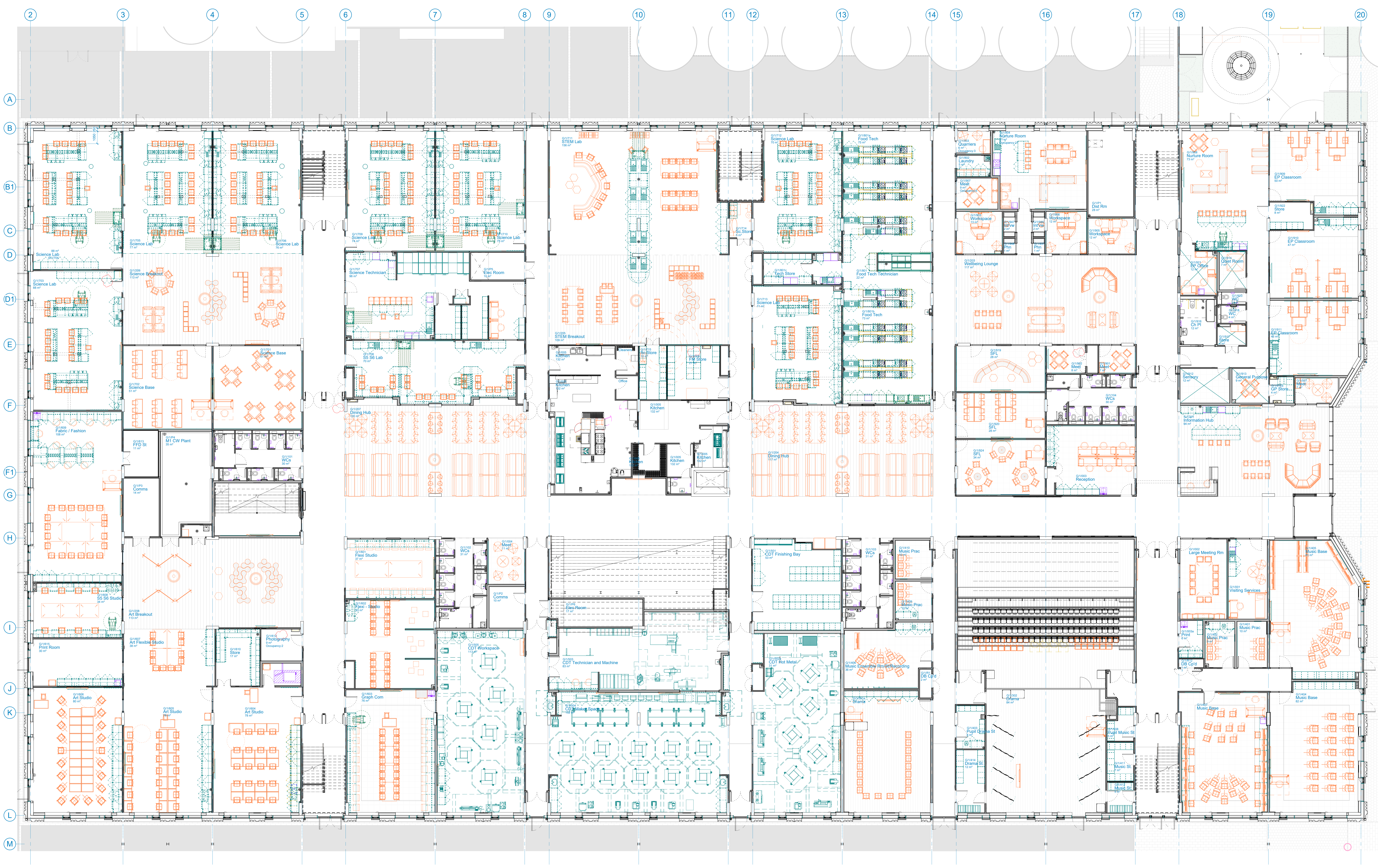
1 Level 0 - Fitout A0 1 : 100
